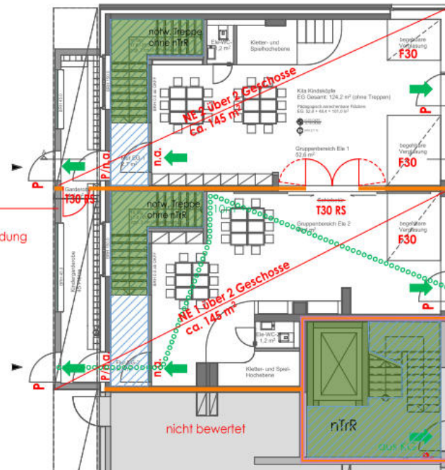
Grundriss Erdgeschoss
