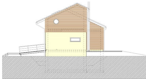
Ansicht Nord-Ost
