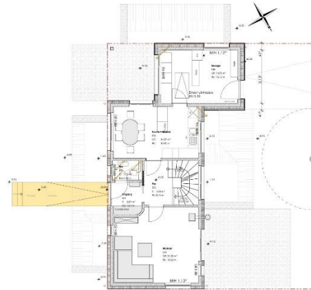
Erdgeschoss
